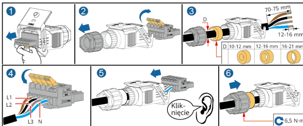
Rysunek 5-8 Przewód czterożyłowy (L1, L2, L3 i N)
