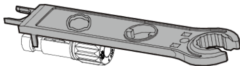
Rysunek 5-15 Odtwarzanie złączy DC
