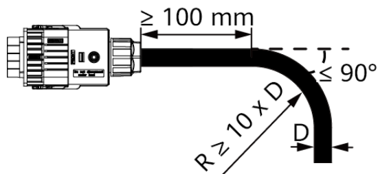
Rysunek 5-11 Poprowadzenie przewodu
