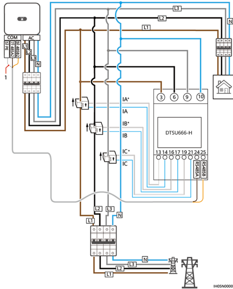
Rysunek 5-25 Połączenie trójfazowe, czteryżytowe (połączenie sieciowe klucza Smart Dongle)
