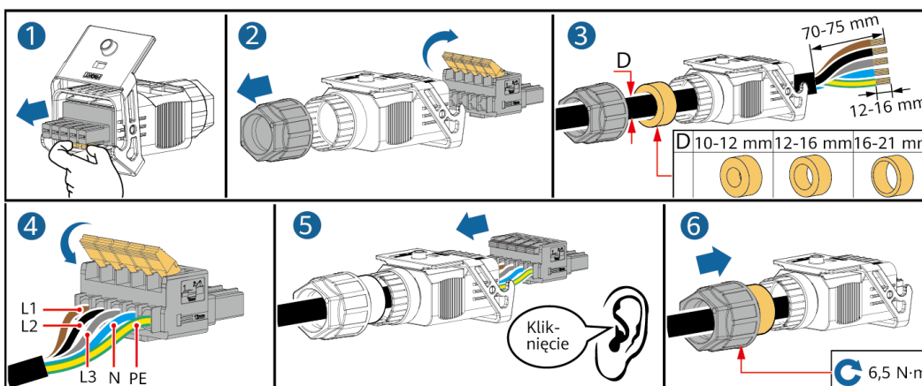
Rysunek 5-9 Przewód pięciożyłowy (L1, L2, L3, N i PE)
