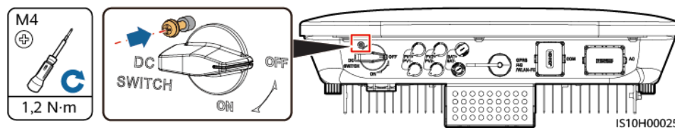
Rysunek 4-10 Przykręcanie śruby zabezpieczającej przelącznika prądu stałego
