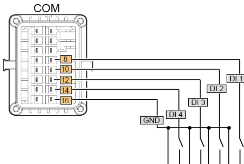
Rysunek 5-34 Połączenie przewodowe
