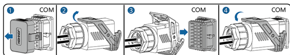
Rysunek 5-23 Podłączanie złącza przewodu sygnałowego
