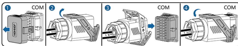
Rysunek 5-31 Podłączenie złącza przewodu sygnałowego
