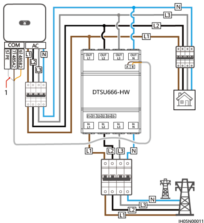
Rysunek 5-27 Bezpośrednie połączenie trójfazowe, czteryżytowe (połączenie sieciowe klucza Smart Dongle)
