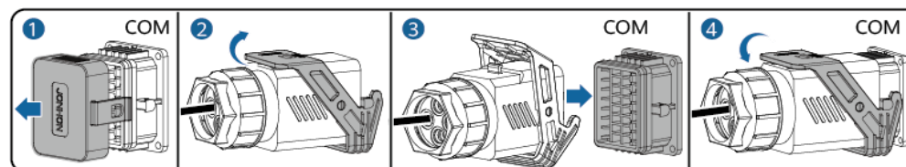
Rysunek 5-36 Podłączanie złącza przewodu sygnałowego
