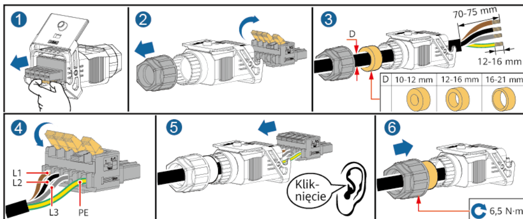
Rysunek 5-7 Przewód czterożyłowy (L1, L2, L3 i PE)
