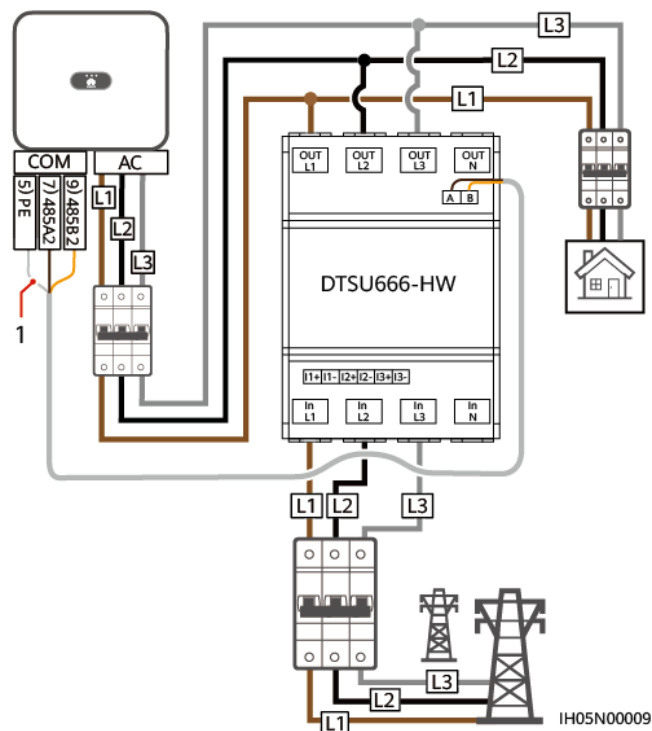
Rysunek 5-26 Bezpośrednie połączenie trójfazowe, trójżytowe (połączenie sieciowe klucza Smart Dongle)
