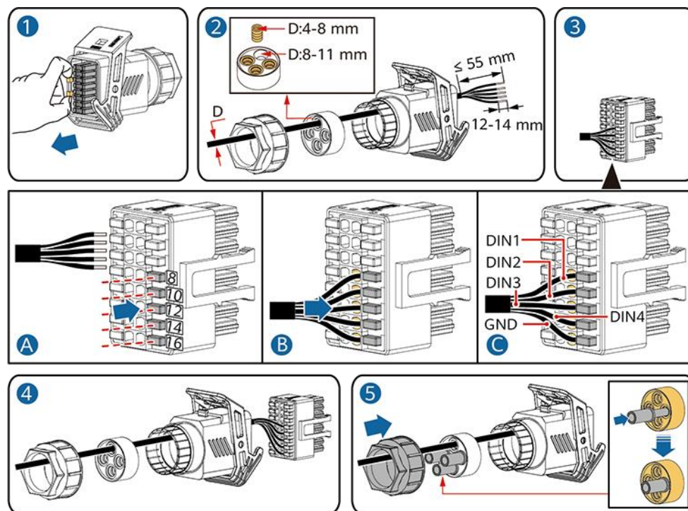
Rysunek 5-35 Instalacja przewodu
