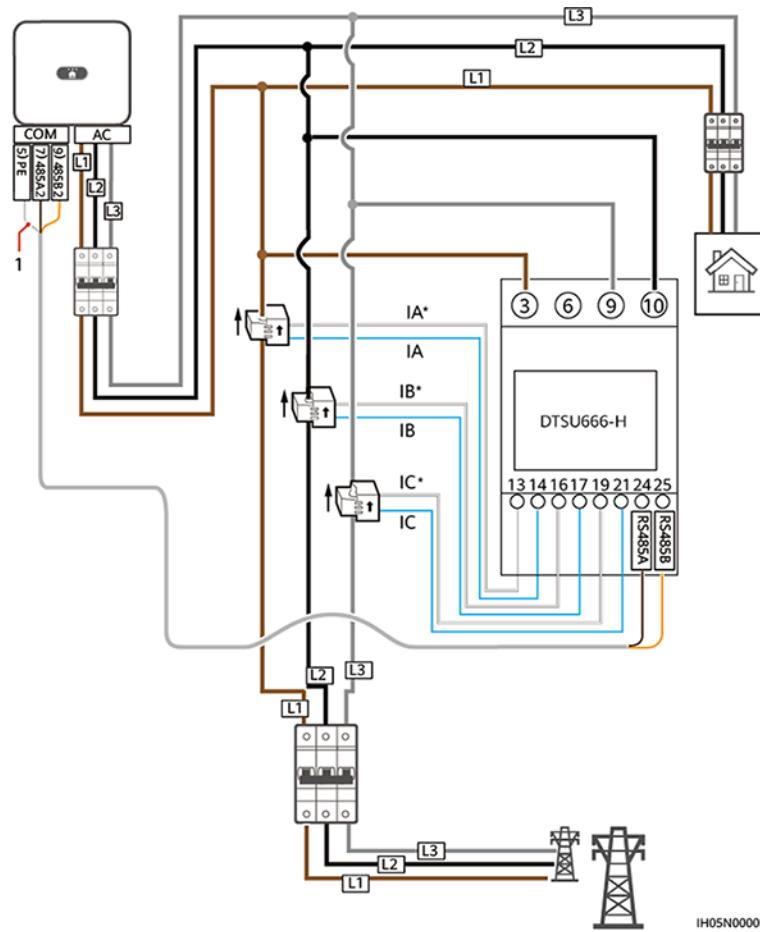
Rysunek 5-24 Połączenie trójfazowe, trójżyłowe (połączenie sieciowe klucza Smart Dongle)
